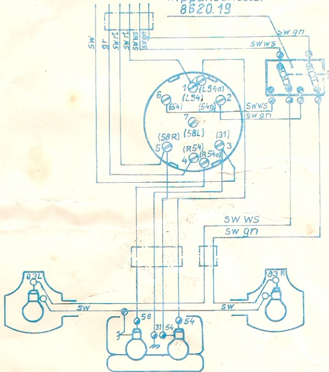
Schaltplan für Anhängerbetrieb (Zugfahrzeug)
